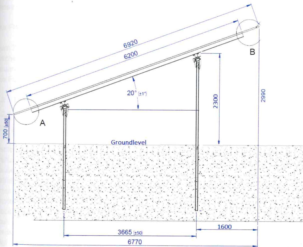
Abb. 7: Schnitt Modultisch
